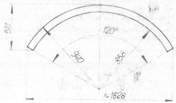
Wymiary segmentów poz 1
