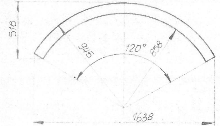
Wymiary segmentów poz 1
